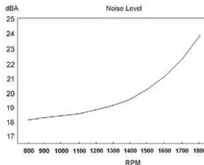
REX-AP750A14 ファンノイズレベル
