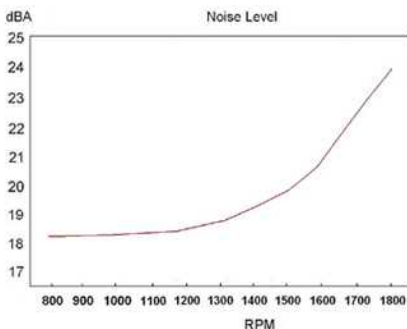
REX-AP650A14 ファンノイズレベル
