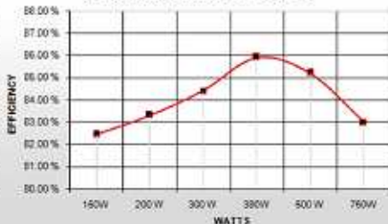
REX-AP750A14 BRONZE 変換効率表
