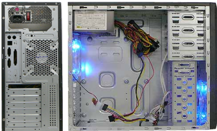
ケース側面 ケースファンは前・にブルーに光ります!
